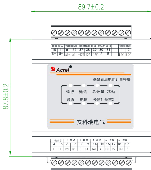
模块主视图
