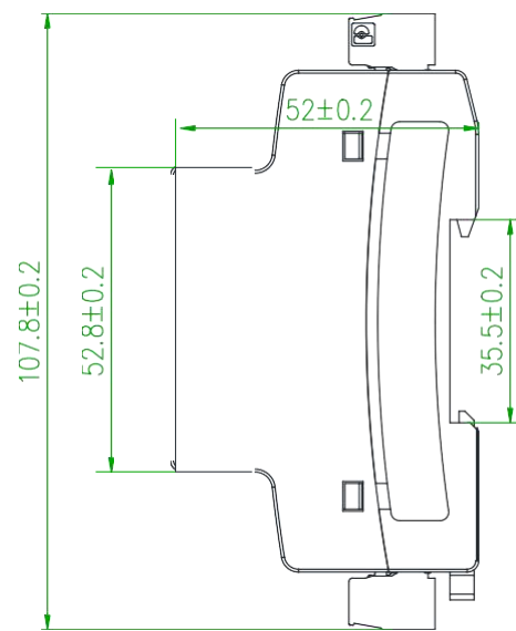
模块左视图
